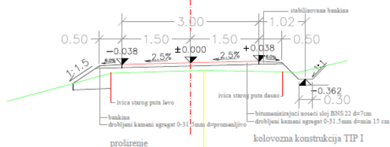
PROFIL "A"
