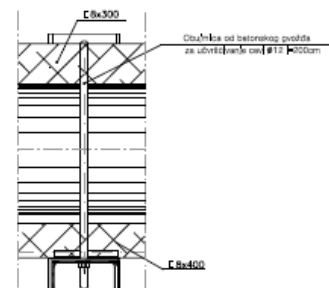
PRESEK 2-2
