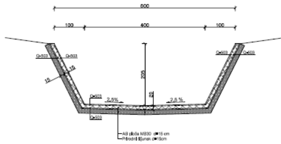
PRESEK A-A BETONSKA REGULACIJA REKE (50m uzvodno | nizvodno)
