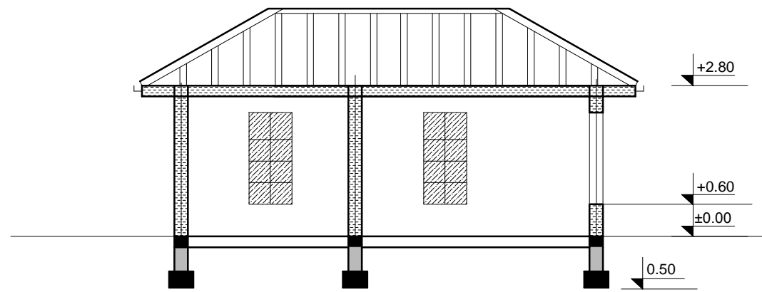
ПРЕСЕК 1 - 1
