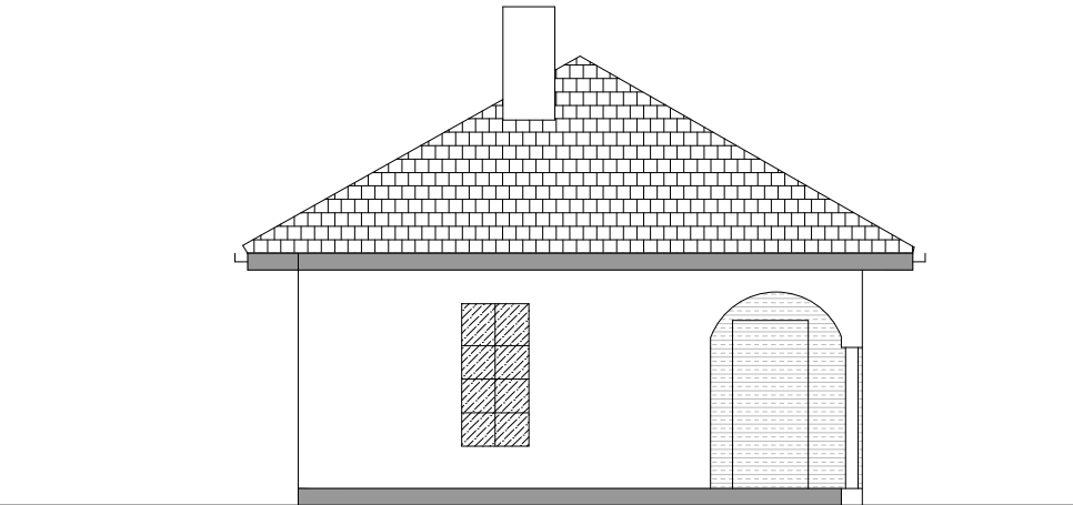
ИЗГЛЕД 3 - 3
