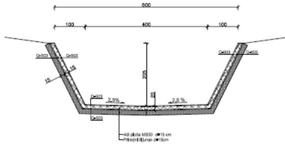
PRESEK A-A BETONSKA REGULACIJA REKE (50m uzvodno | nizvodno)
