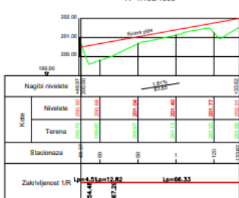
ПОДУЖНИ ПРОФИЛ ЗИДА 0+049.97-0+133.62 R=1:100/1000
