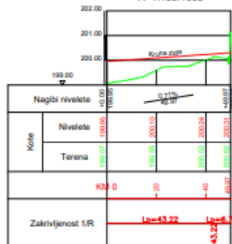
ПОДУЖНИ ПРОФИЛ ЗИДА 0+000-0+049,97 R=1:100/1000
