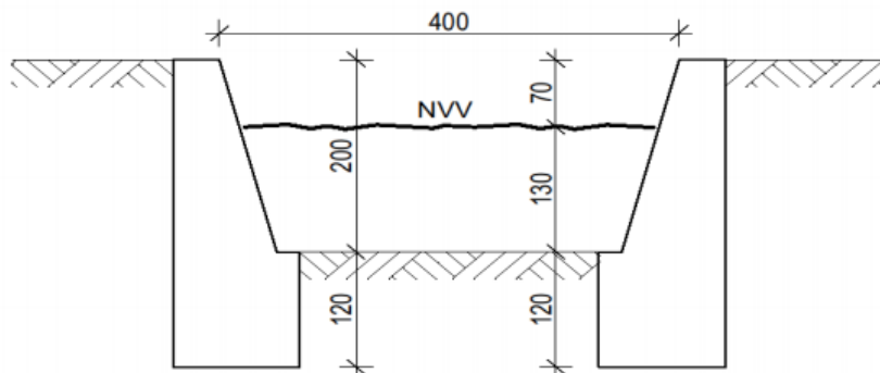
Попречни профил Смиловачке реке
