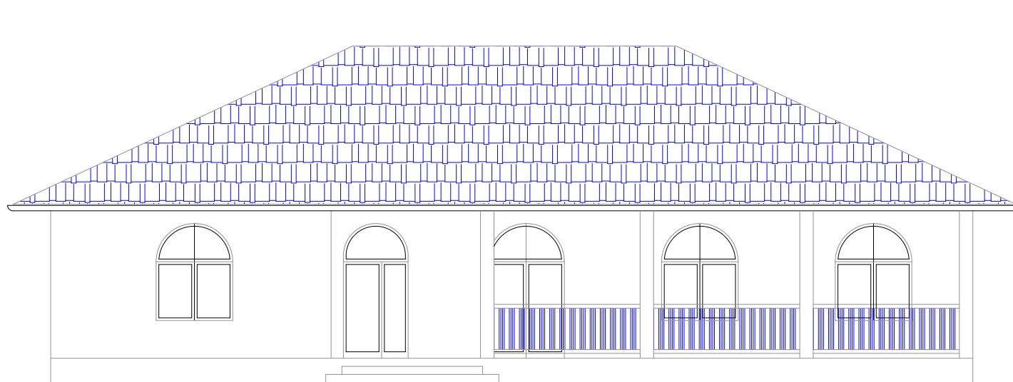
JUŽNI IZGLED
